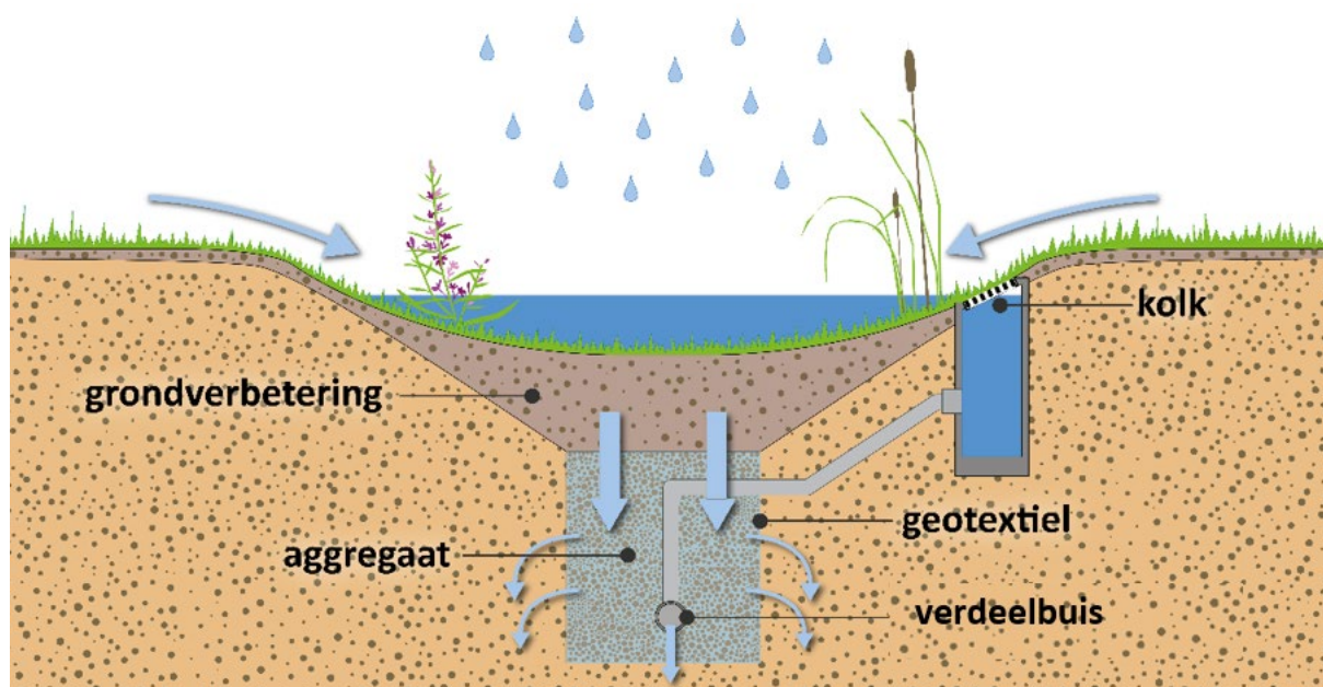
Opbouw van een wadi (Blauwgroenvlaanderen.be)
