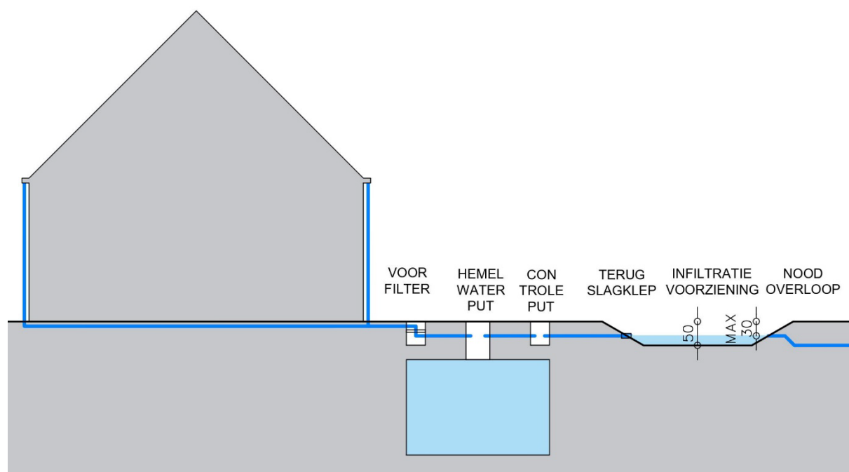
Afbeelding: ter plaatse gemetste voorfilter
