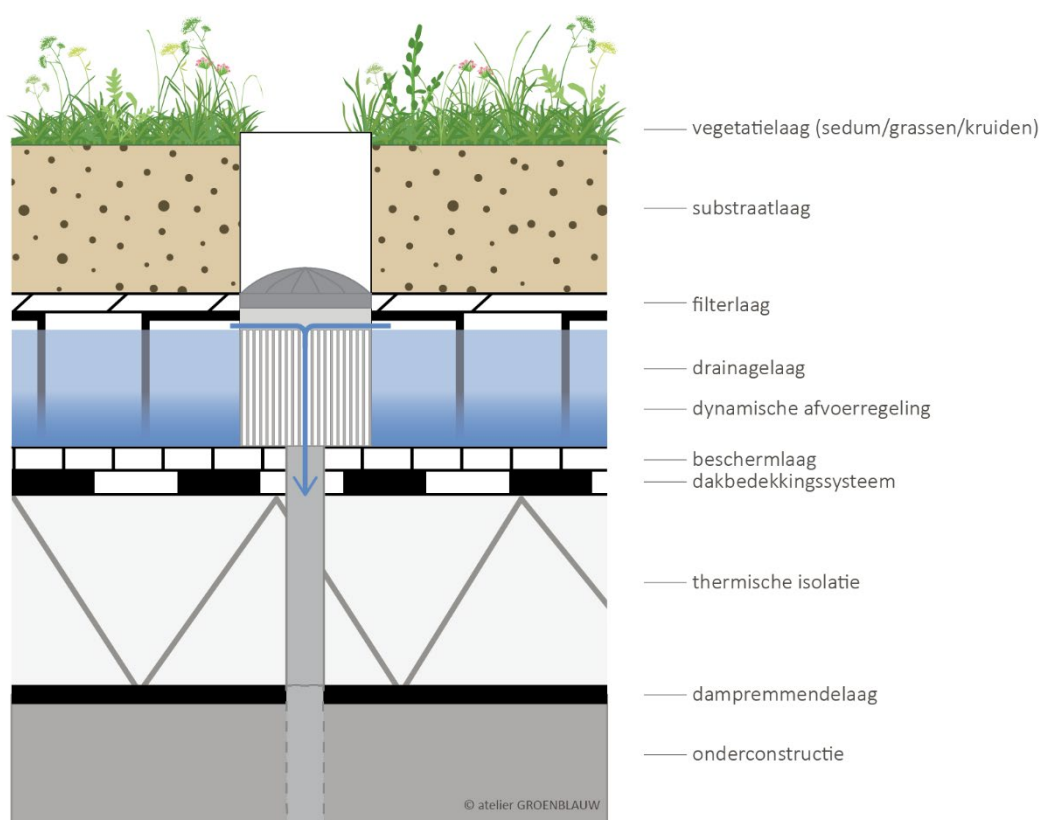
Afbeelding: Retentiedak van Blauwgroenvlaanderen.be
