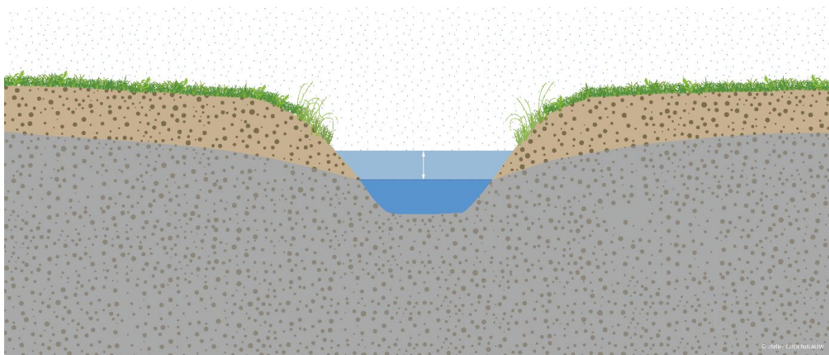
Opbouw van een infiltratiegracht (Blauwgroenvlaanderen.be)
