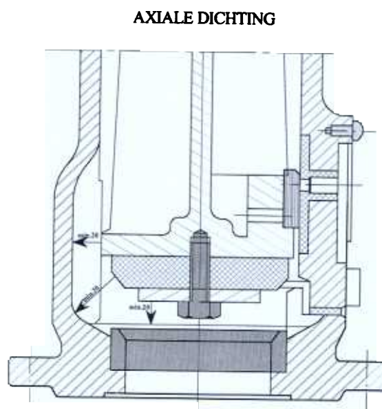
principetekening 3
