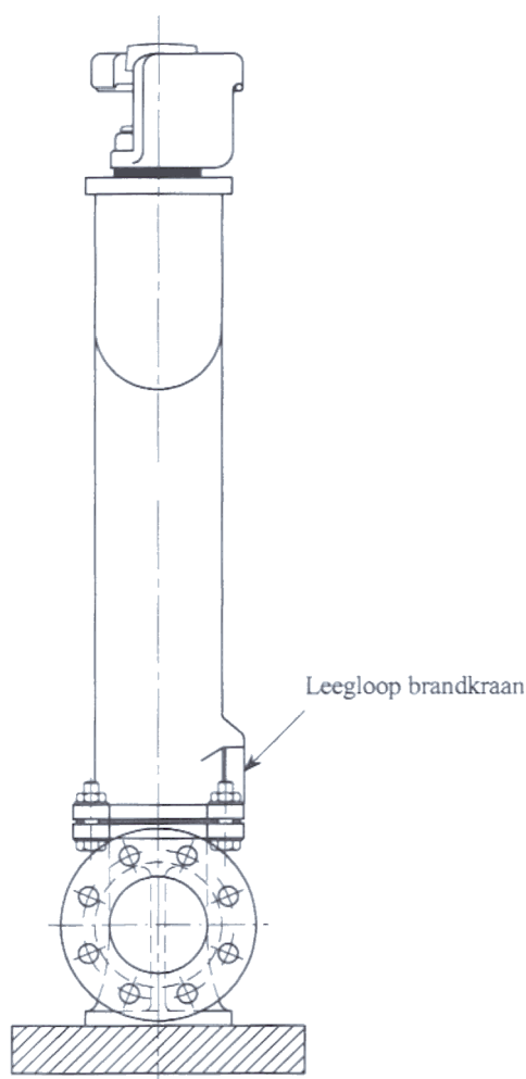
Tekening 5
