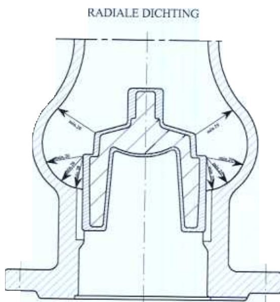
principetekening 2
