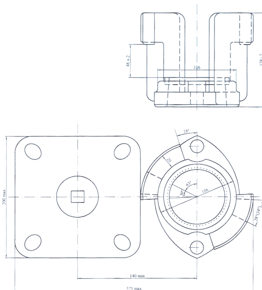
tekening 4
