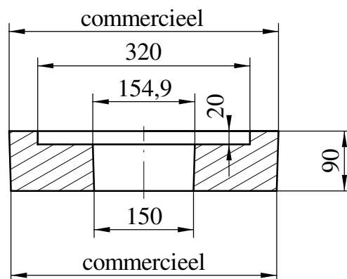
Snede A-B
