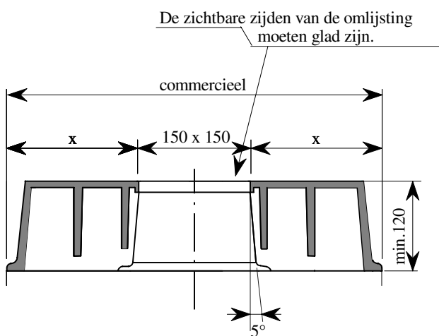
Snede A-B
