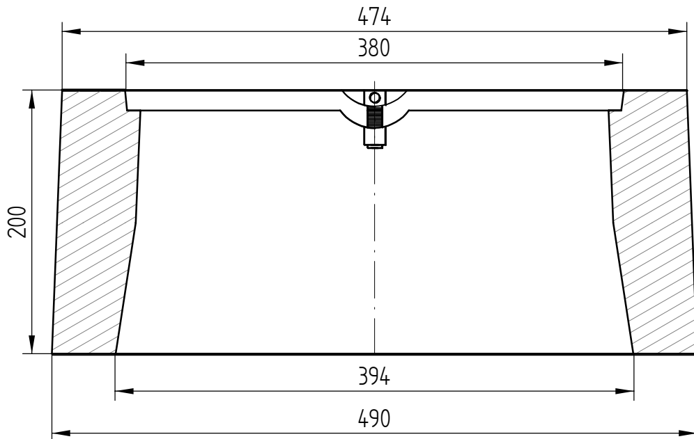
Snede A-B
