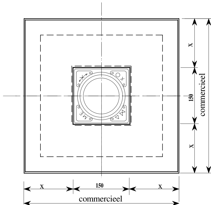
Bovenaanzicht
